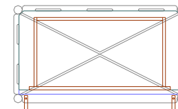
Schubkasten-Element ② auf tiefengekürztem Einlegeboden *nur in Verbindung mit Schubkasten-Element ① oder Schubkasten-Element ③
